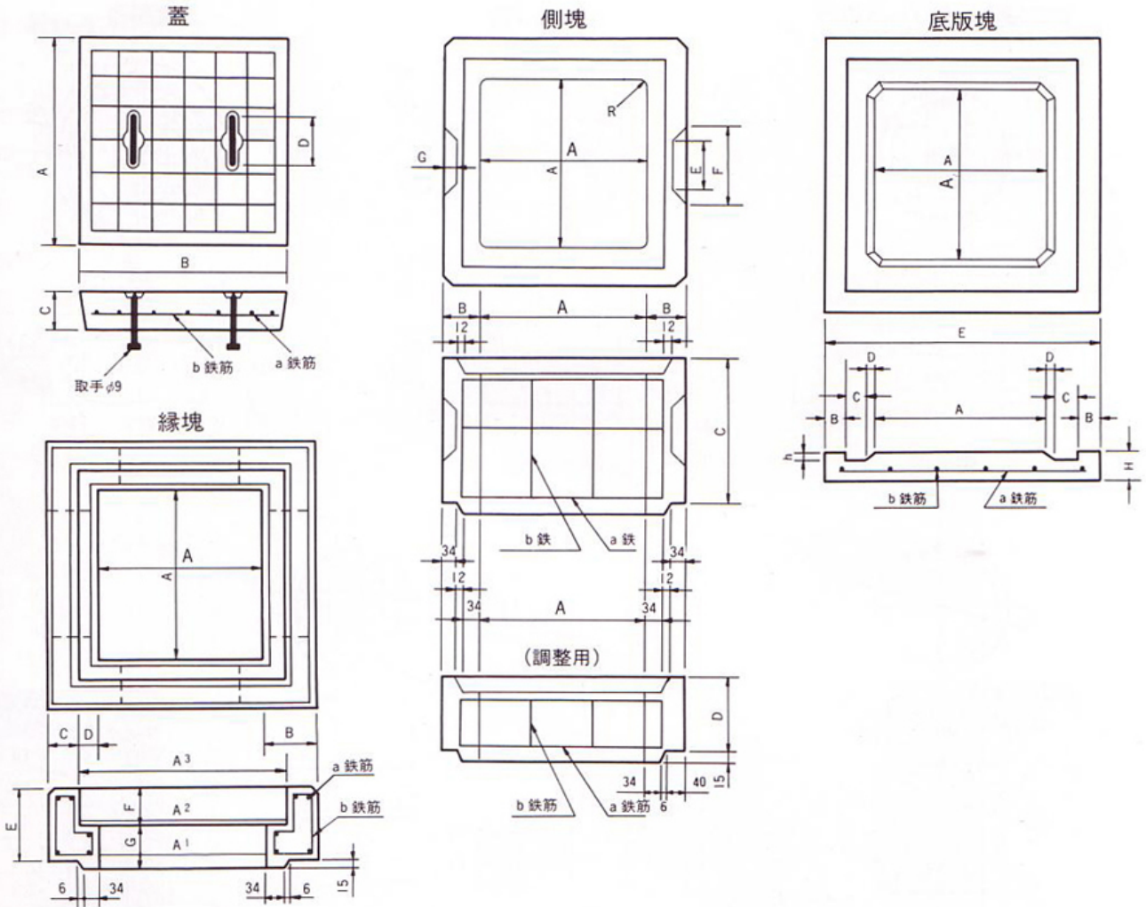
形状・寸法及び配筋
