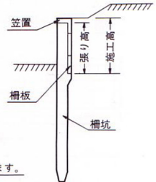
一般組立図
