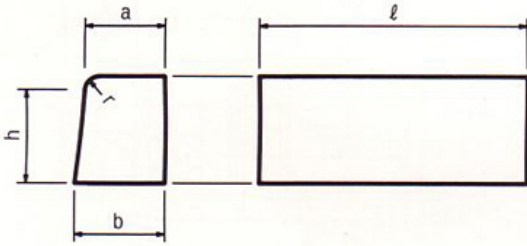
片面歩車道境界ブロック
