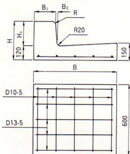
形状・寸法及び配筋
