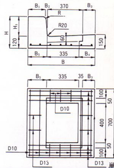
形状・寸法及び配筋
