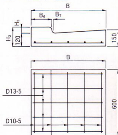
形状・寸法及び配筋
