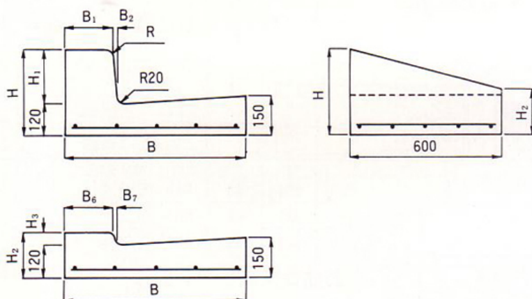
形状・寸法及び配筋
